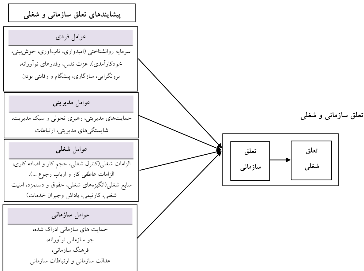
شکل ۱- مدل مفهومی پژوهش (محقق ساخته)
