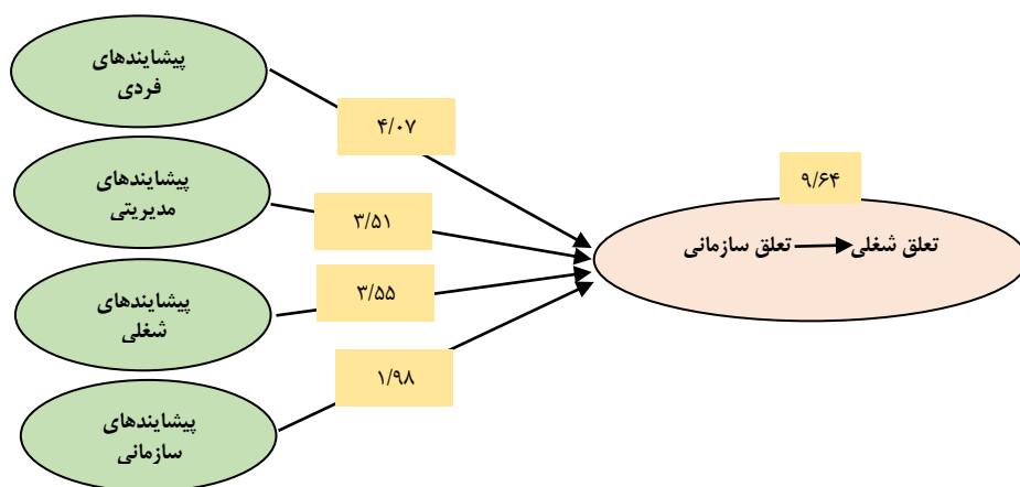
شکل ۳- مدل اندازه‌گیری پژوهش در حالت معناداری
